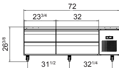
MGF8463GR
