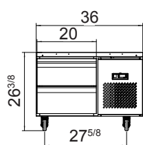
MGF8458GR
