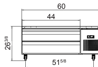
MGF8462GR
